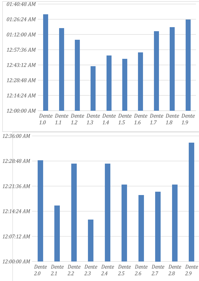
Gráfico 5 – Tempo de execução utilizando a FCC.
